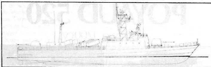
Patrouilleur rapide lance-missiles Combattante III B de 395 tonnes, construit par CNM (France) ; la version tunisienne sera légèrement différente de ce qui est indiqué sur ce croquis ; elle comportera, entre autres équipements, 8 missiles mer-mer Exocet et deux canons de 30 mm Oerlikon
